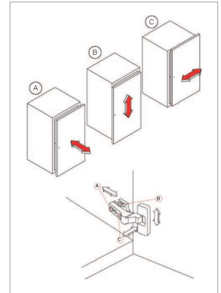
Beschläge: Dreifach verstellbare Scharniere
